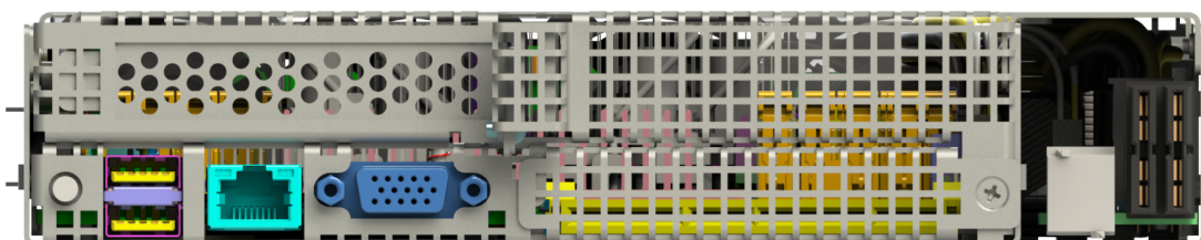
Модуль вычислительный «Тип2» / Вид сзади
