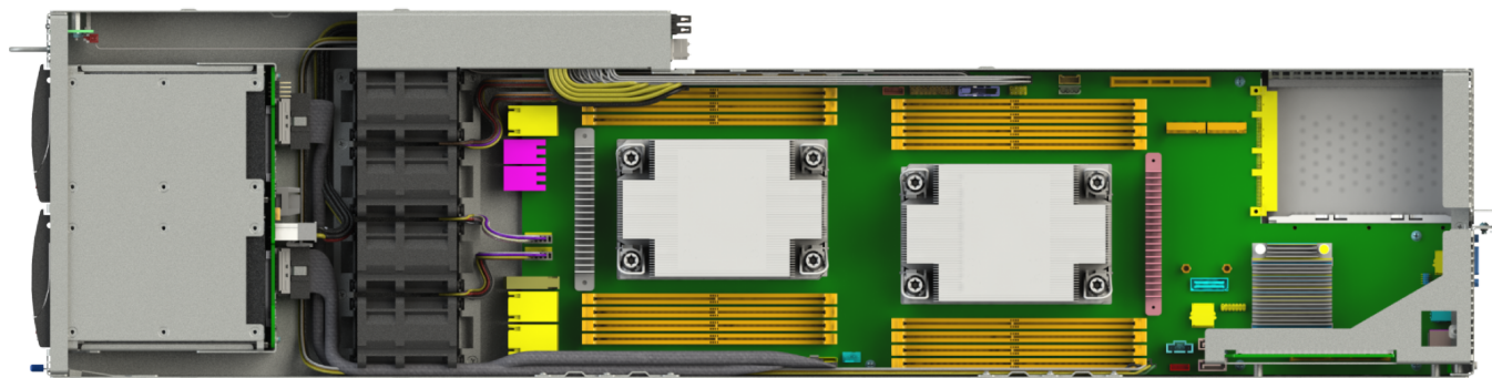
Модуль вычислительный «Тип2» / Вид сверху
