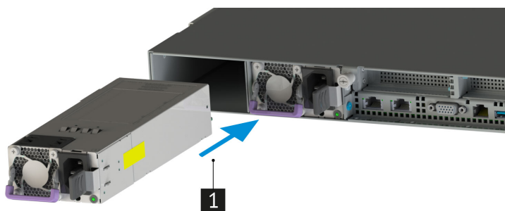
Рис. 52. Установка блока питания
