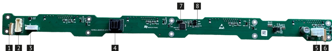
Рис. 13. Плата расширения 4LFF (НИКА.469535.070)
