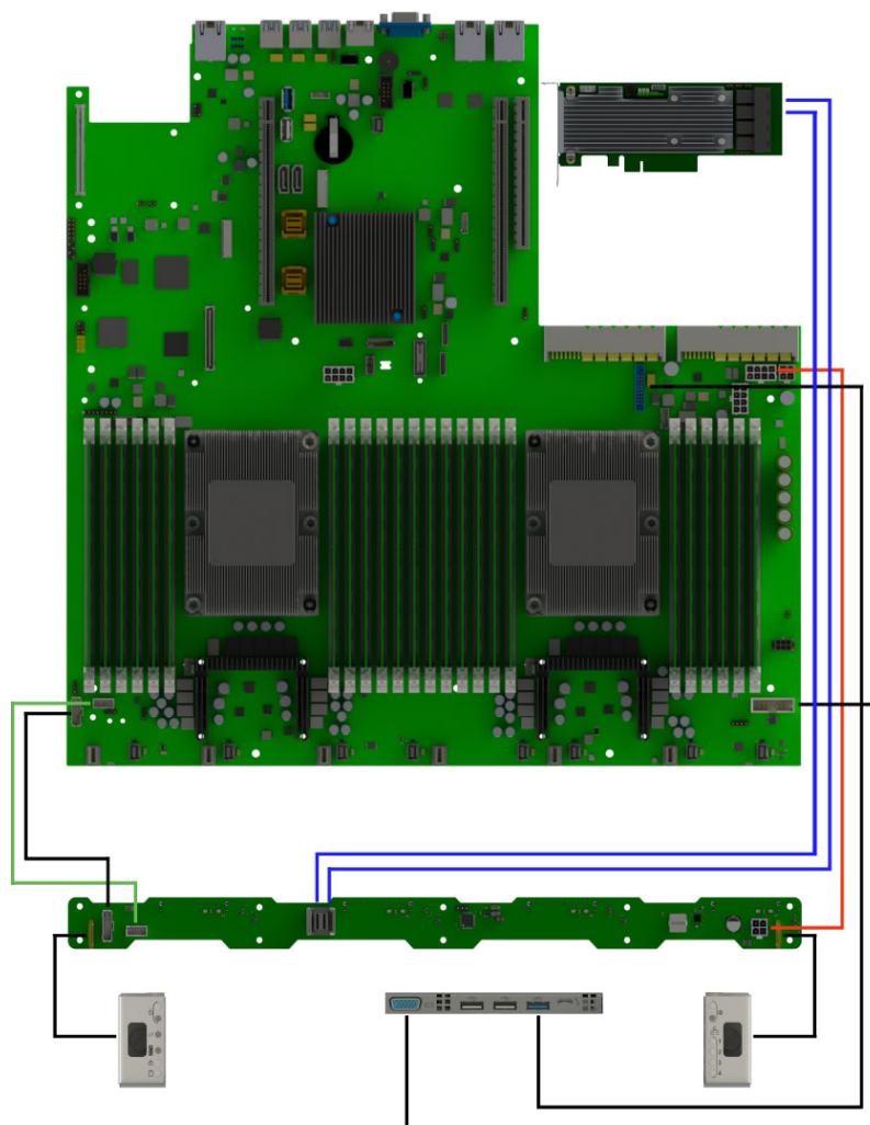
Рис. 27. Схема прокладки системных кабелей и кабелей питания с подключением PCIe RAID
