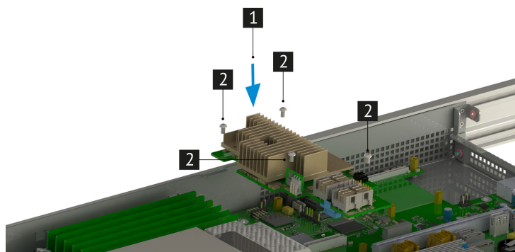
Рис. 44. Установка наплатного RAID-контроллера
