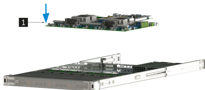
Рис. 39. Установка материнской платы
