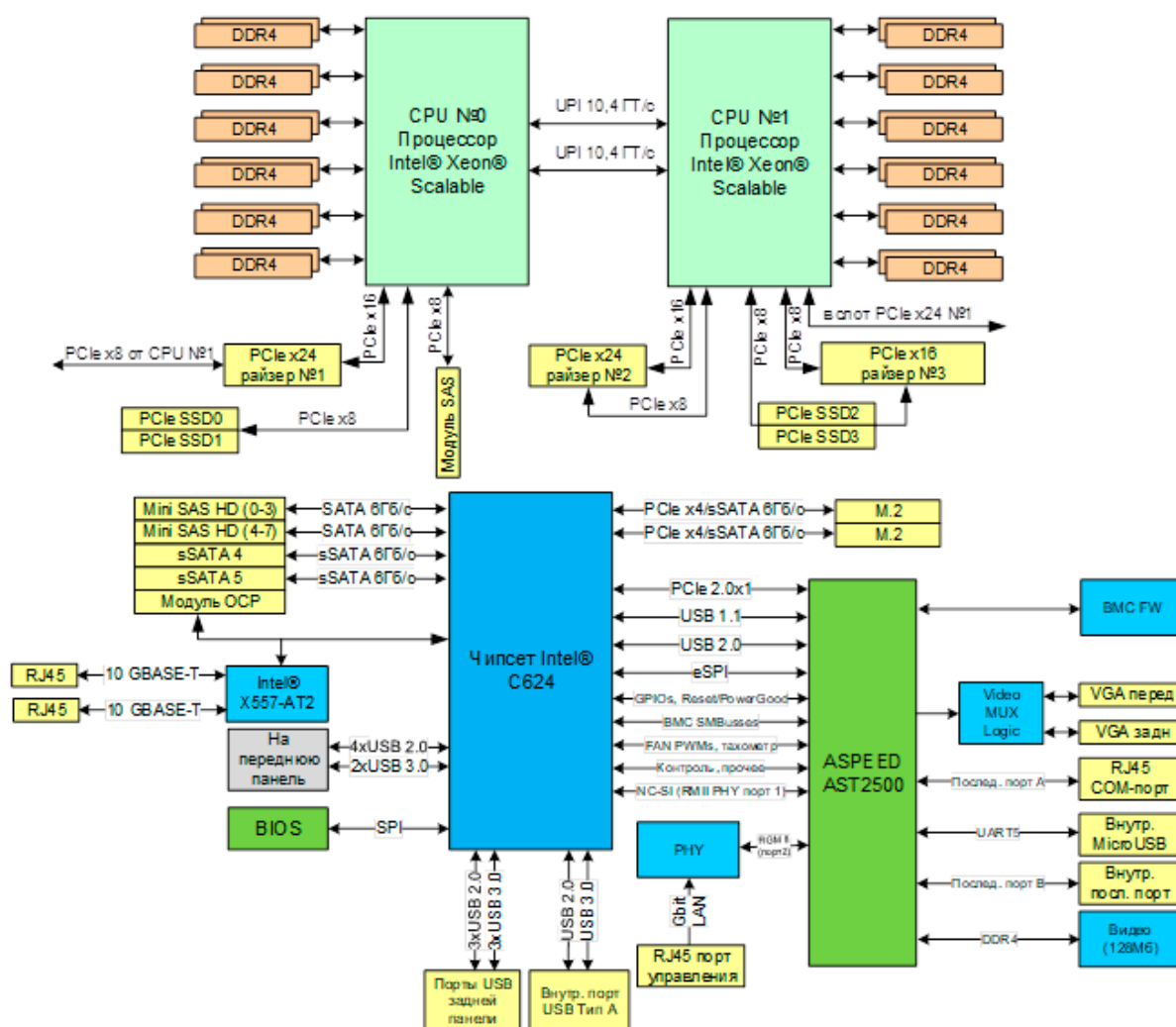
Рис. 1. Структурная схема материнской платы НИКА.469555.001
