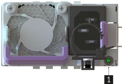
Рис. 48. Светодиодная индикация состояния блока питания
