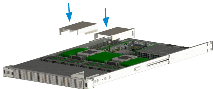
Рис. 23. Установка воздушного кожуха
