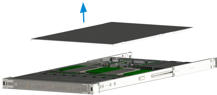
Рис. 20. Снятие верхней крышки платформы
