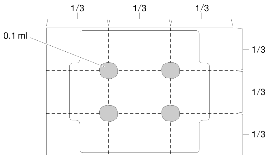
Рис. 36. Нанесение термопасты
