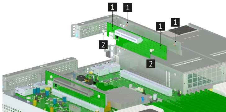
Рис. 45. Установка PCIe-райзера на основании
