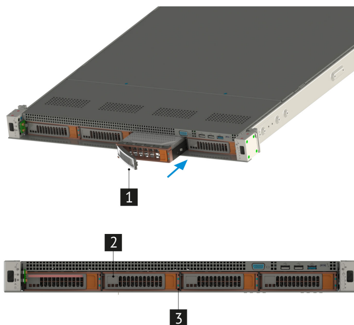
Рис. 42. Извлечение дисков
