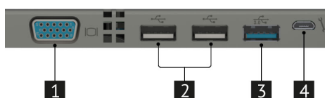
Рис. 5. Передняя панель
