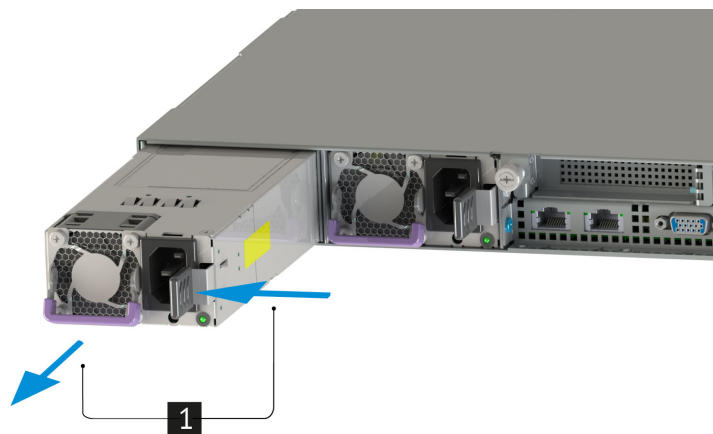
Рис. 49. Извлечение блока питания
