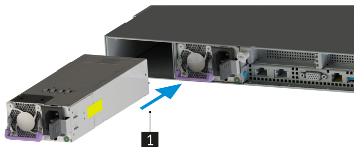
Рис. 50. Установка блока питания
