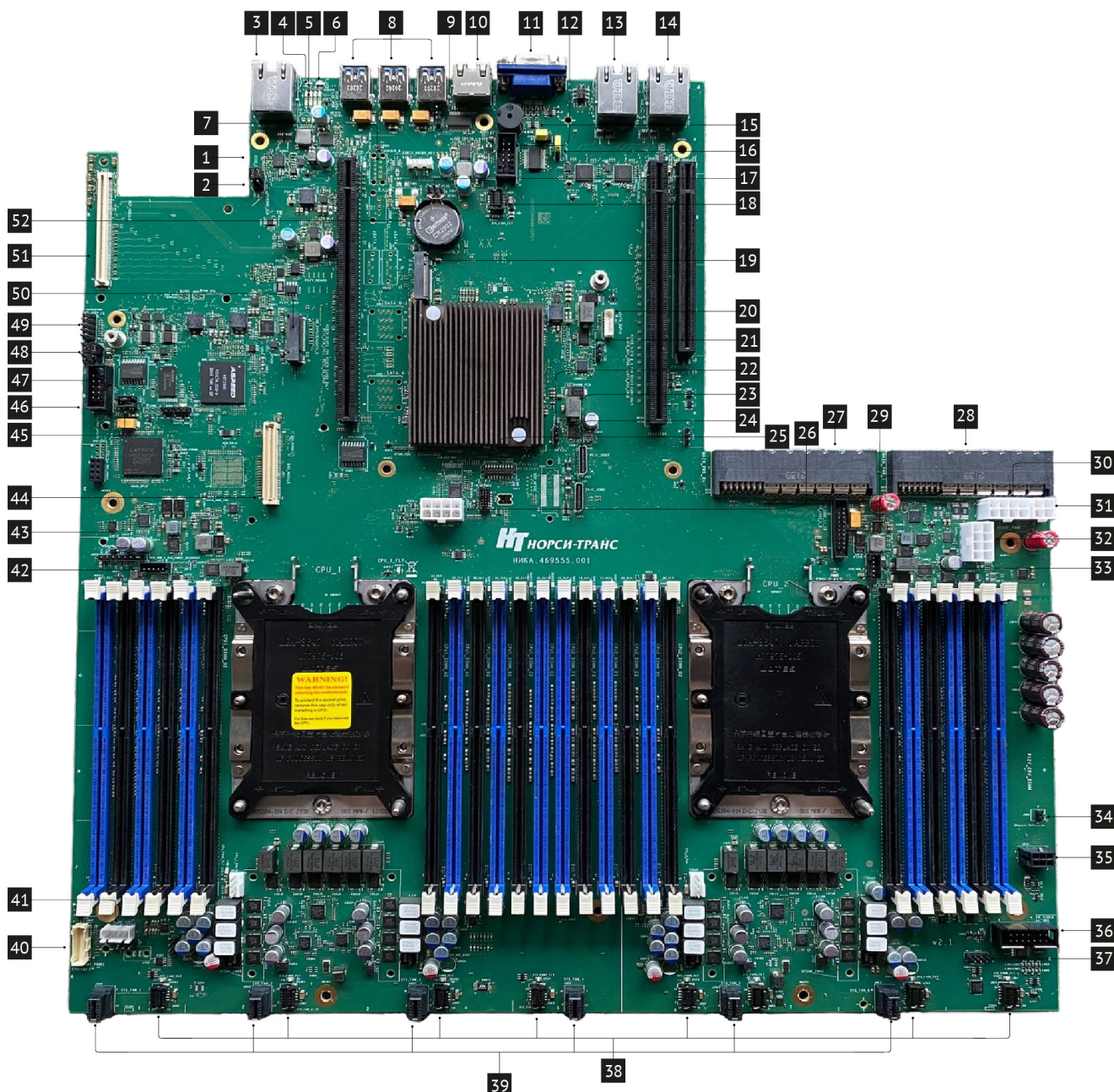
Рис. 12. Соединители и переключатели материнской платы
