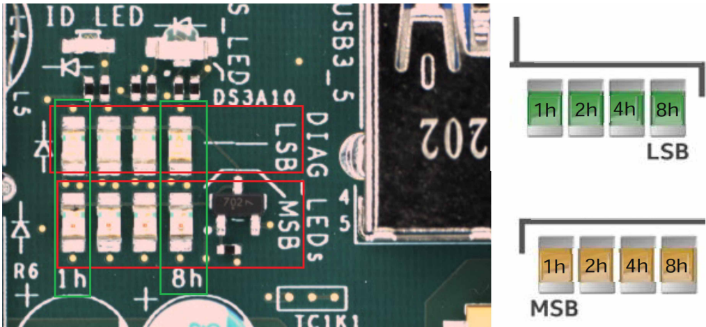
Рис. 8. Расположение и определение POST CODE LED
