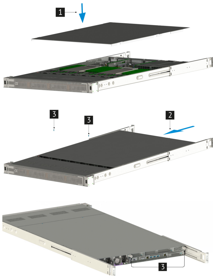
Рис. 21. Установка верхней крышки платформы
