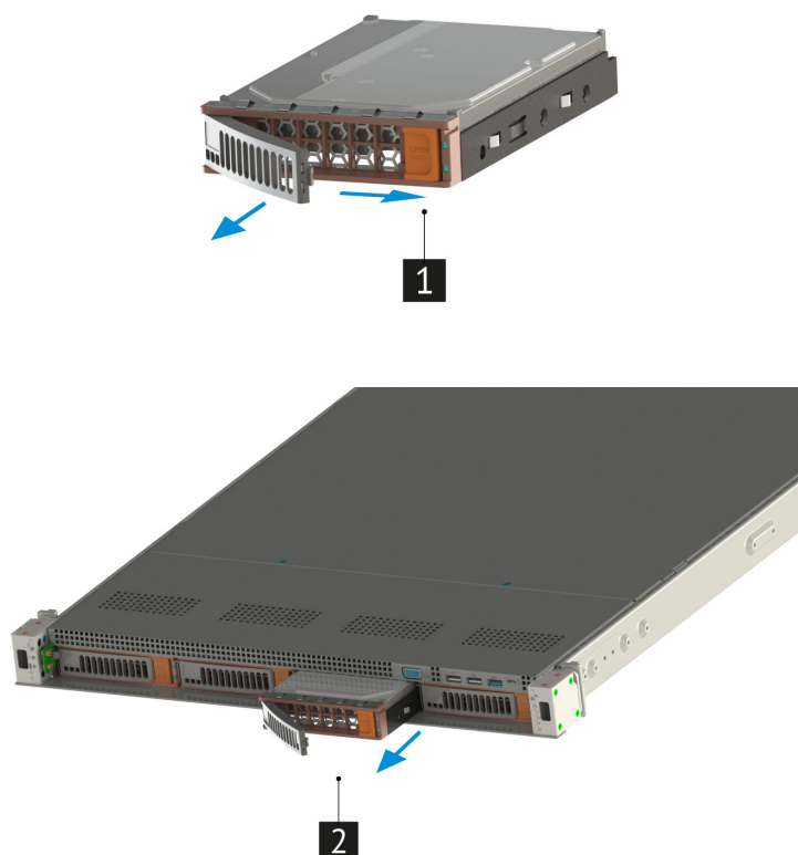
Рис. 41. Извлечение дисков
