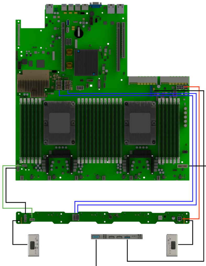
Рис. 26. Схема прокладки системных кабелей и кабелей питания с подключением наплатного RAID
