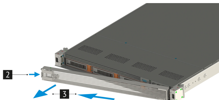
Рис. 17. Снятие передней панели
