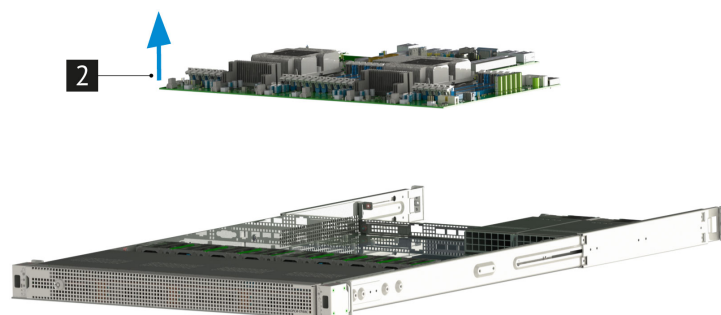
Рис. 38. Извлечение материнской платы
