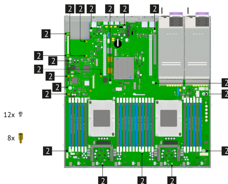
Рис. 40. Винты и стойки фиксирующие материнскую плату
