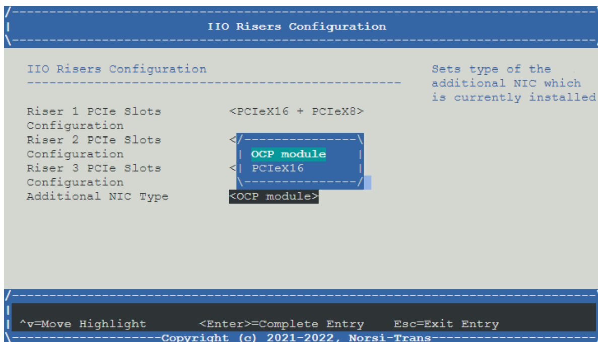
Рис. 64. Меню IIO Risers Configuration
