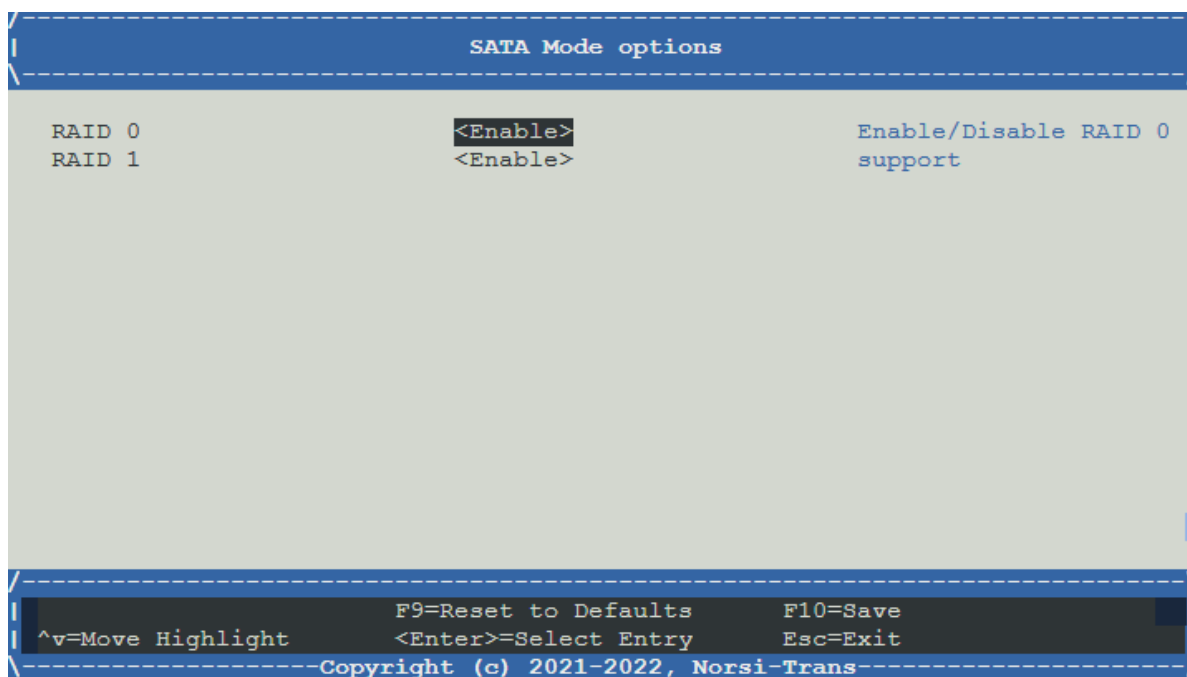
Рис. 60. Меню SATA Mode option
