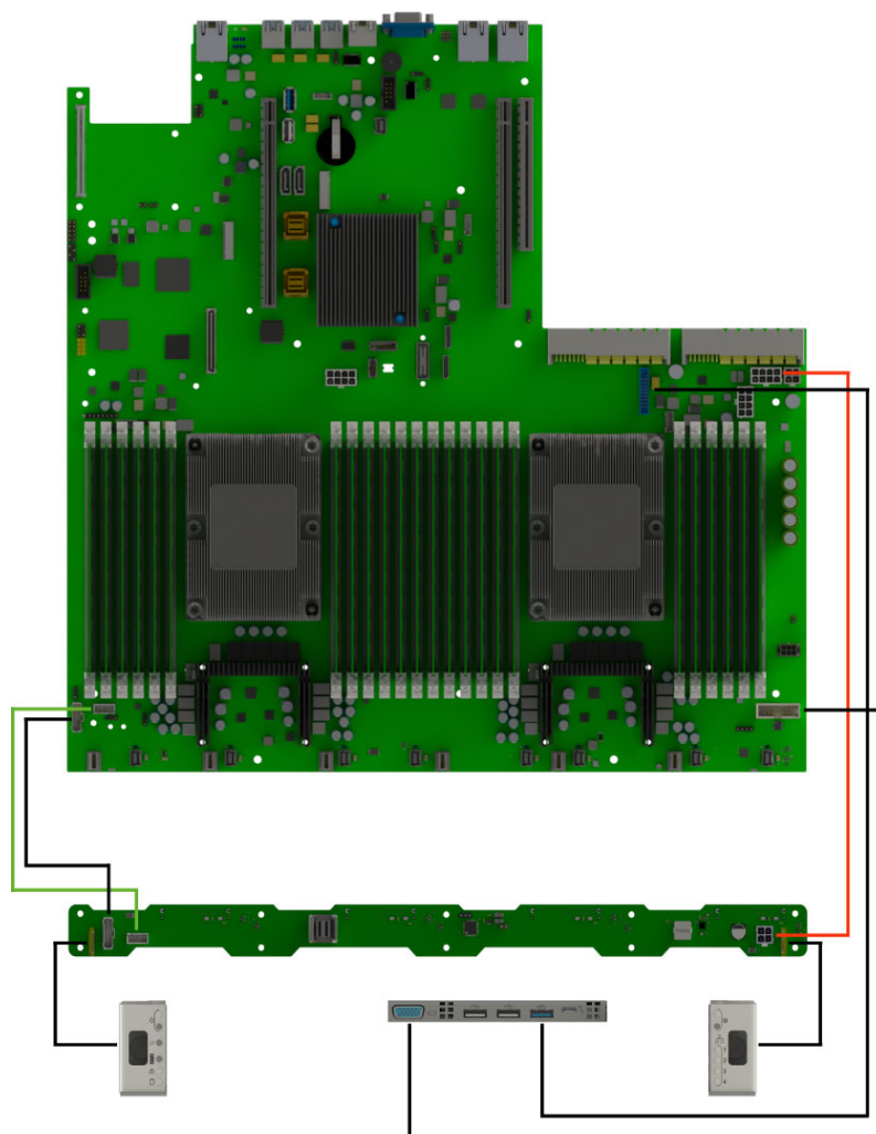
Рис. 25. Схема прокладки системных кабелей и кабелей питания
