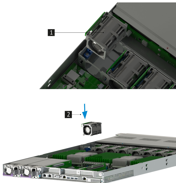
Рис. 29. Подключение вентилятора
