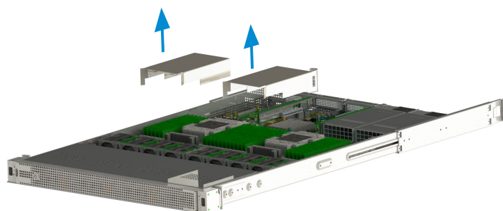
Рис. 22. Снятие воздушного кожуха
