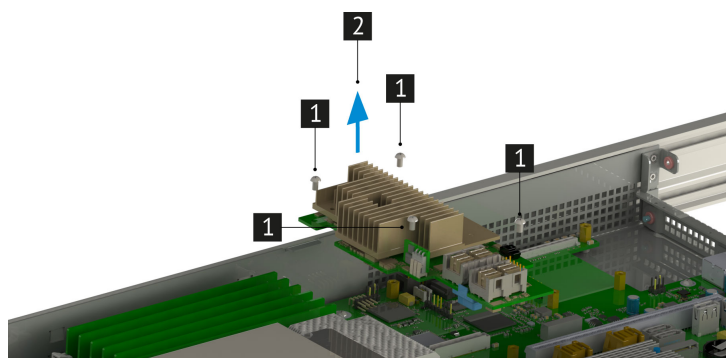
Рис. 43. Снятие наплатного RAID-контроллера
