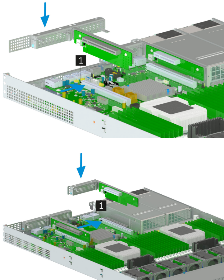
Рис. 46. Установка PCIe-райзера с основанием в корпус сервера
