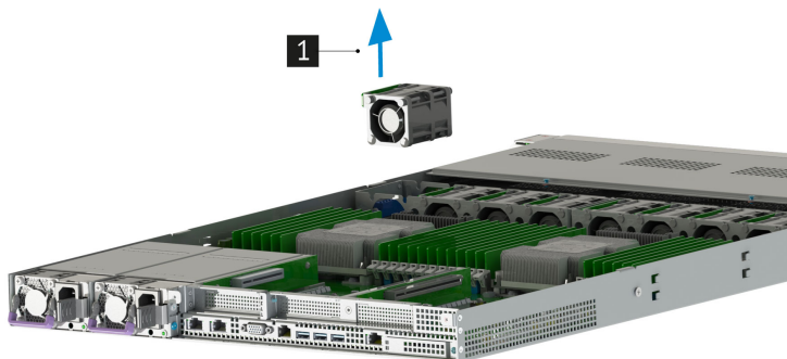
Рис. 28. Извлечение вентилятора
