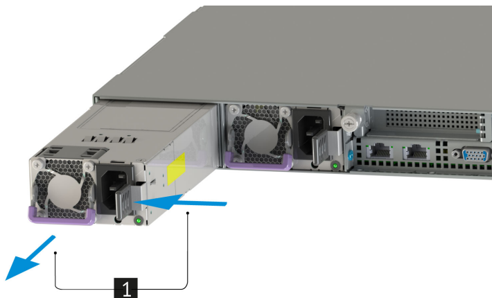
Рис. 51. Извлечение блока питания
