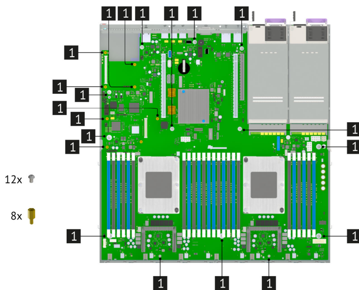
Рис. 37. Винты и стойки фиксирующие материнскую плату
