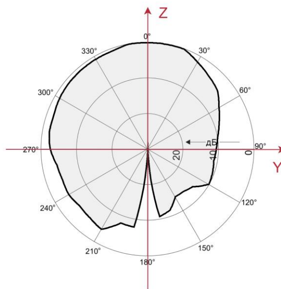
Вертикальная (угломестная)
