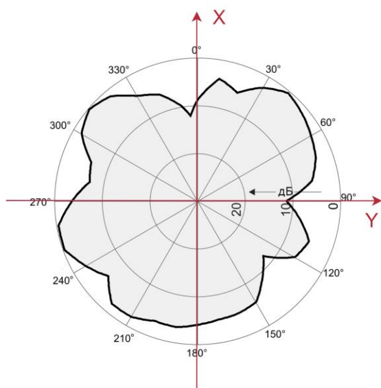
Горизонтальная (азимутальная)
