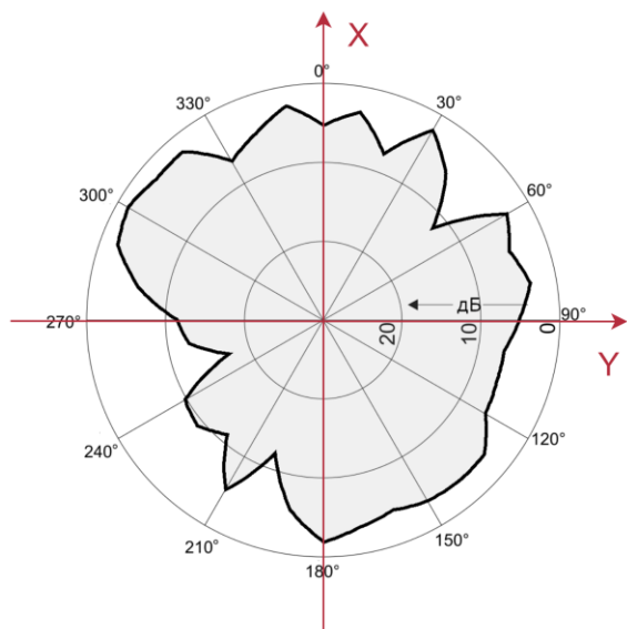
Горизонтальная (азимутальная)
