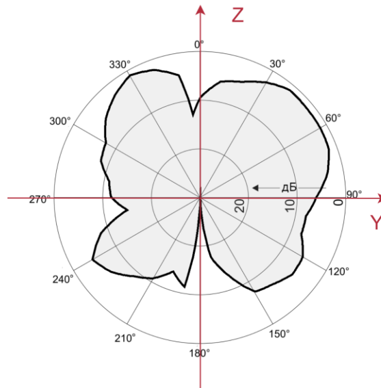
Вертикальная (угломестная)
